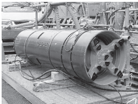
▲推進工法(小口径)
